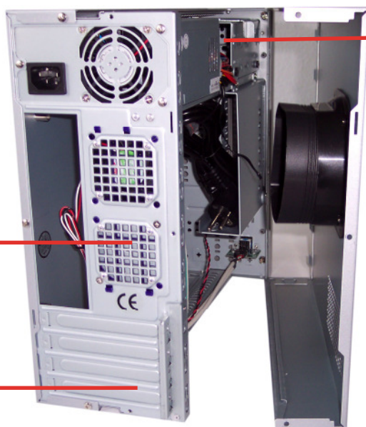
Festplattenkäfing
