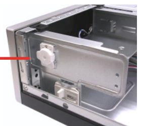
Schraubenlose HDD, ODD Assemblierung
